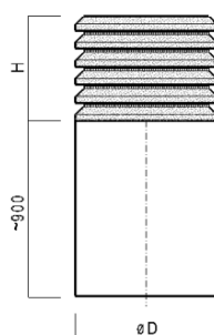
Ausführung: Bündig ab ø180
